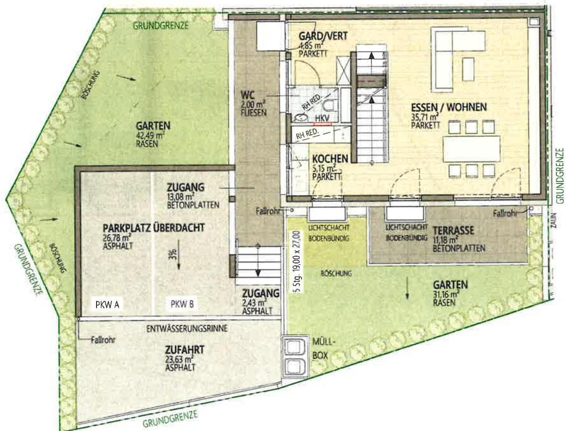
ERDGESCHOSS
