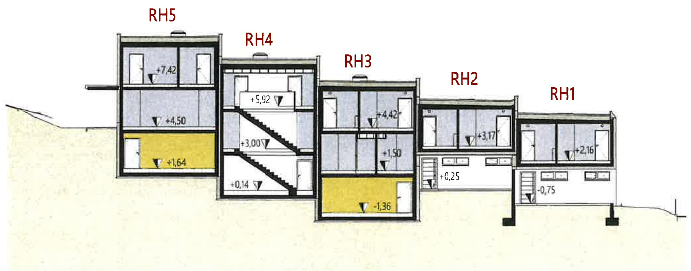
ÜBERSICHTSSCHNITT 1-1
